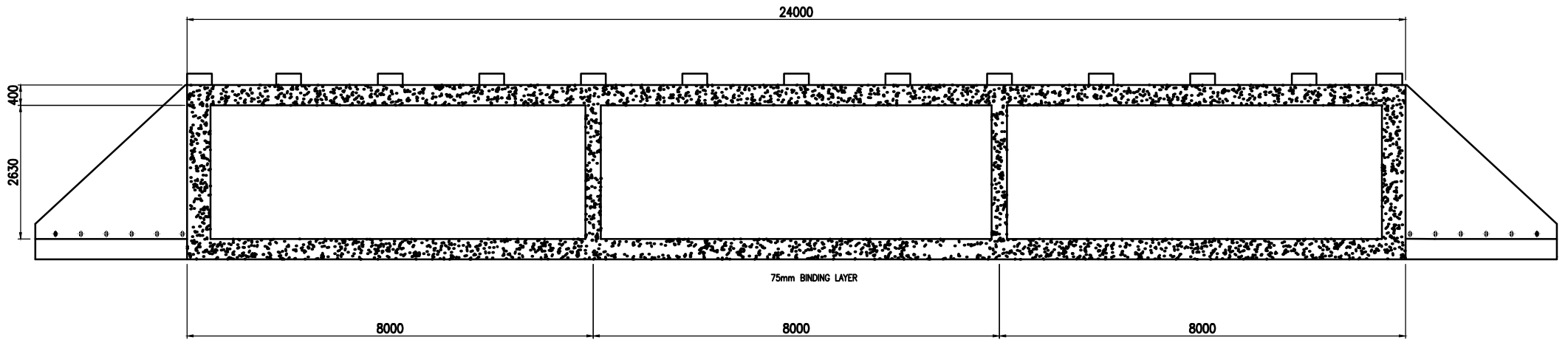
SIDE VIEW A-A SCALE: 1:50
