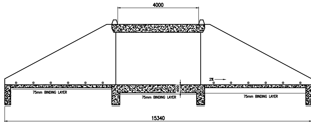
SIDE VIEW B-B SCALE: 1:50
